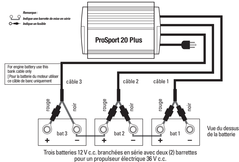
Fig. 3 Chargeur trois bancs ProSport 15 (OEM seulement) et 20 pour 3 batteries 12 V
