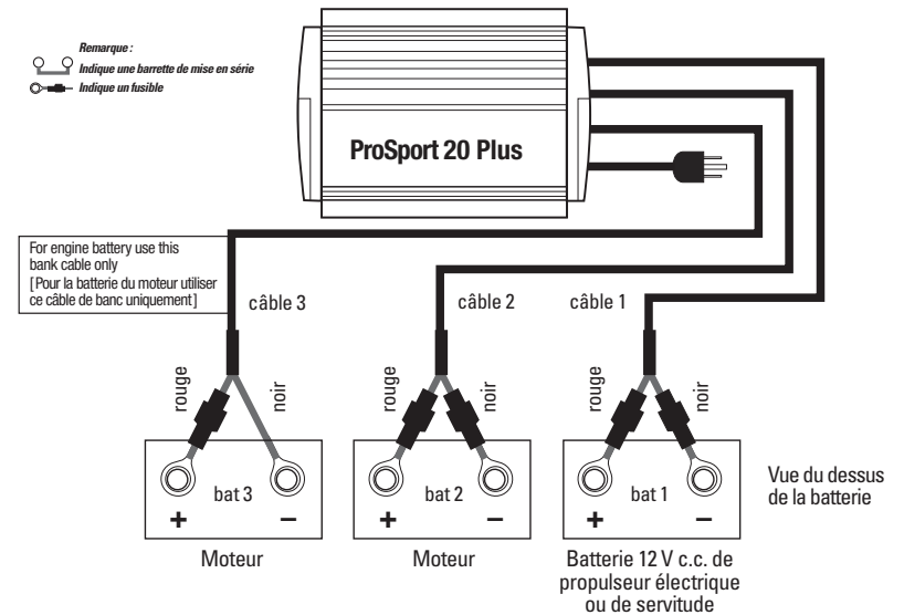
Fig. 1 Chargeur trois bancs ProSport 15 (OEM seulement) et 20 pour 3 batteries 12 V
