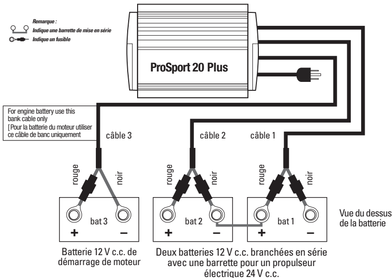
Fig. 2 Chargeur trois bancs ProSport 15 (OEM seulement) et 20 pour 3 batteries 12 V
